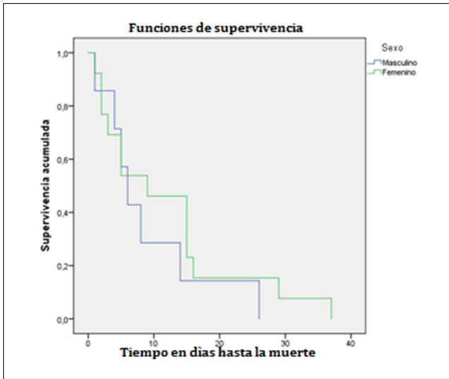
Figura 1. Curva de supervivencia para el tiempo en días entre inicio de síntomas y la muerte de pacientes menores de edad diagnosticados con COVID-19 en Colombia. Método Kaplan Meier.
